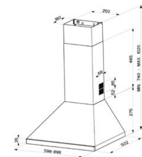
Designkupa Strip 60 och Strip 90 rostfri
